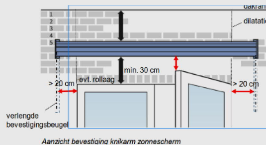
Aanzicht bevestiging knikarm zonnescherm
